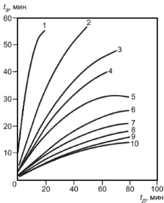
Рисунок Р.5 - Зависимость эквивалентной продолжительности пожара t_3 от продолжительности пожара t_{\text{п}} для горизонтальных незащищенных металлических конструкций
