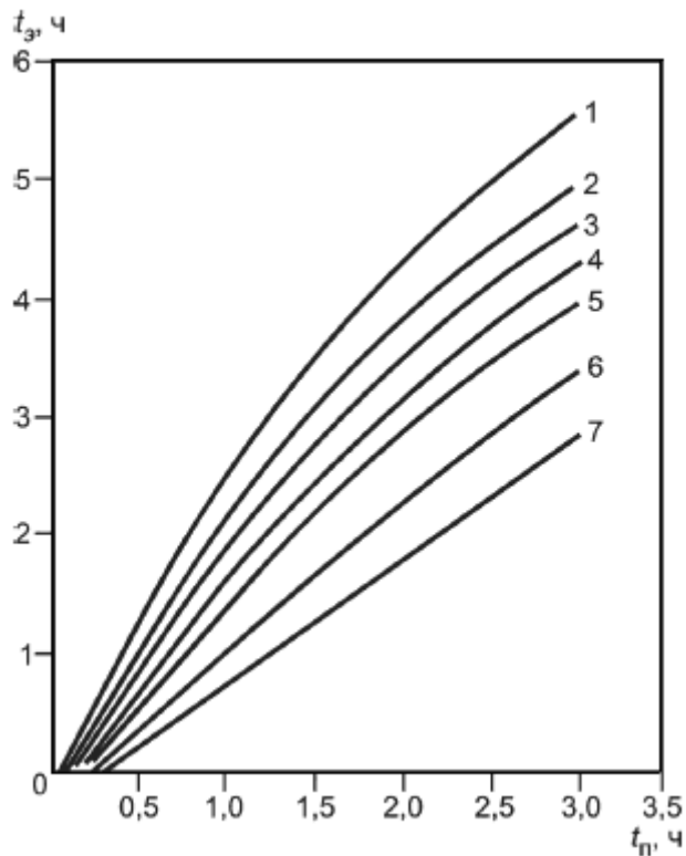
Рисунок Р.9 - Зависимость эквивалентной продолжительности пожара t_3 от характерного времени объемного пожара t_n для центрально сжатых железобетонных колонн
