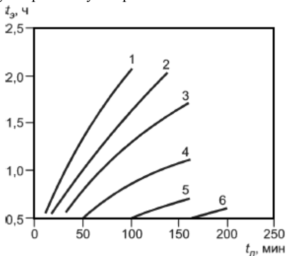
Рисунок Р.4 - Зависимость эквивалентной продолжительности пожара t_3 от продолжительности пожара t_{\text{п}} для железобетонных и огнезащищенных металлических конструкций перекрытия при горении ЛВЖ и ГЖ
